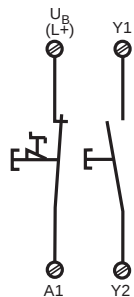
Fig. 5: Circuito de entrada monocanal: conexonado de PARADA DE EMERGENCIA, rearme manual/Circuito di ingresso monocanal: circuito di arresto di emergenza; start manuale/Eenkanalig ingangscircuit: Noodstopschakeling; handmatige start
