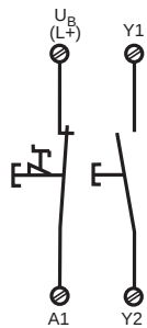
Fig. 5: Eingangskreis einkanalgig: NOT-AUS-Beschaltung; manueller Start/ Single channel input circuit: Emergency Stop wiring; manual reset/ Commande par 1 canal : circuit AU, avec réarmement manuel
