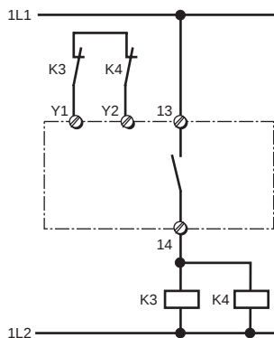
Fig. 6: Refuerzo (multiplicación) de los contactos mediante contactores externos, monocanal, rearme automático/Aumento della portata (del numero) dei contatti mediante relè esterni; monocanal; start automatico/Versterking (vermenigvuldiging) van de contacten via externe magneetschakelaars; eenkanalig; automatische start
