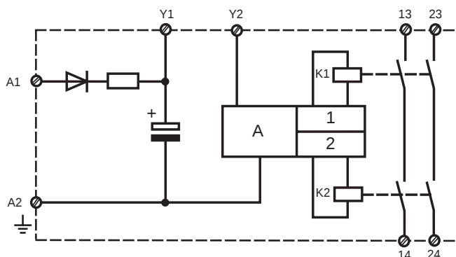
Fig. 1: PNOZ X7P 24 V DC/AC - Plano de conexiones esquemático/Schema di collegamento/Intern schema
