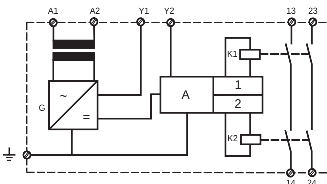
Fig. 2: PNOZ X7P AC - Plano de conexiones esquemático/Schema di collegamento/Intern schema
